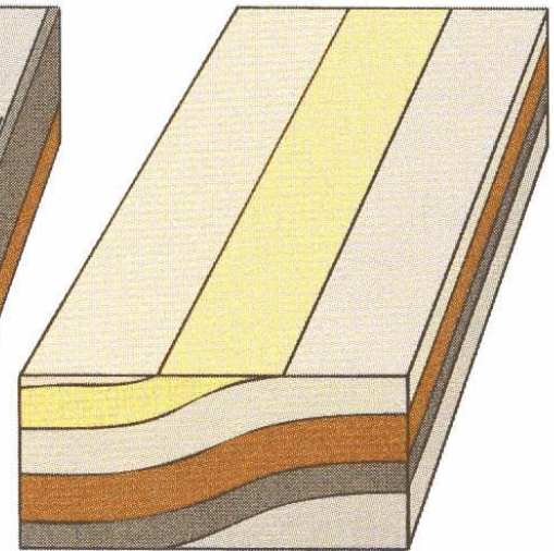
Monocline
