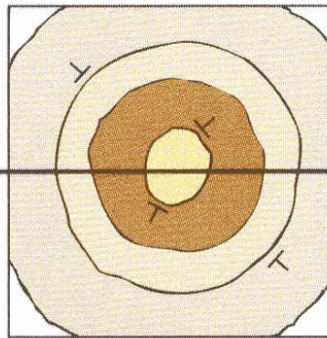
Dome
